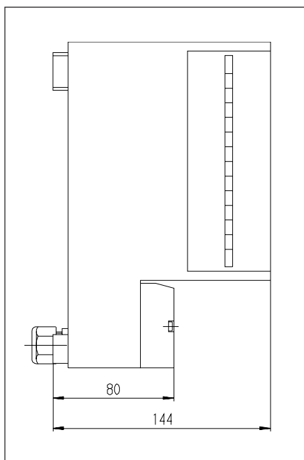
Skříňka monitoru
